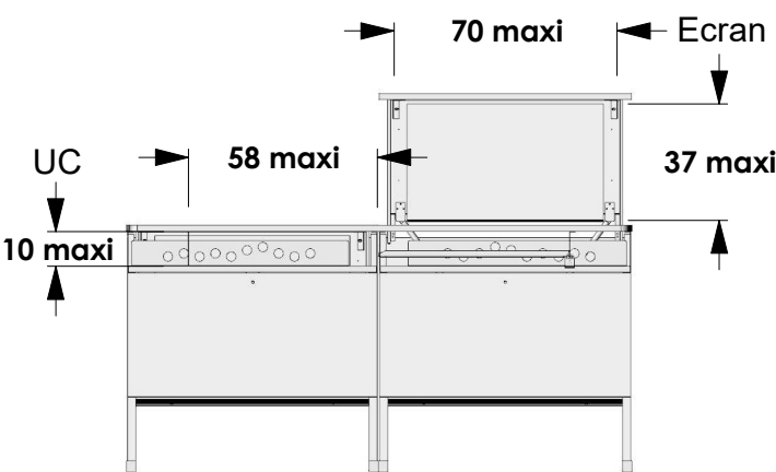
vue face
